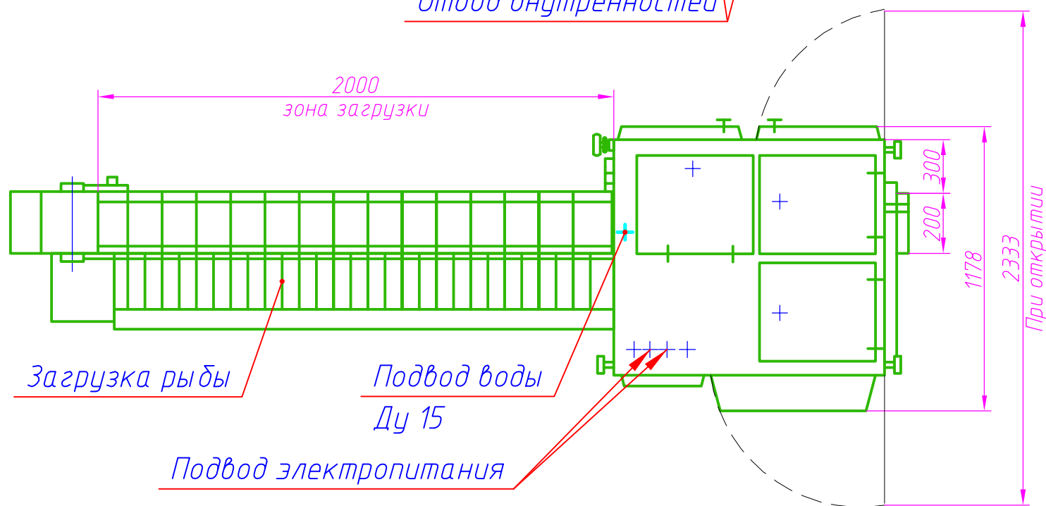
Схема расположения фундаментных болтов
